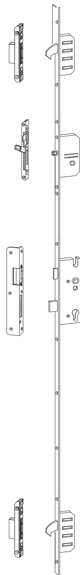
M2-W 3 - fach Verriegelung mit 2 Haken und Türspaltsicherung Farbe Topzink
