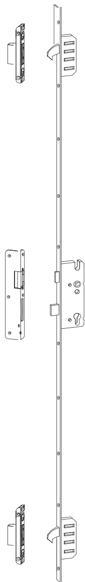
M2 3 - fach Verriegelung mit 2 Haken Farbe Topzink (Standard)
