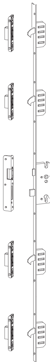
M4 5 - fach Verriegelung mit 4 Haken Farbe Topzink
